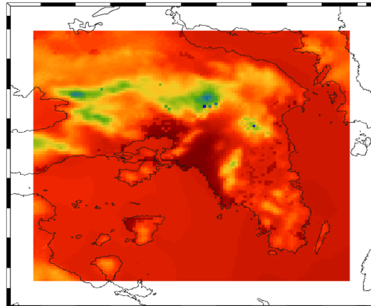
WRF 1x1km
