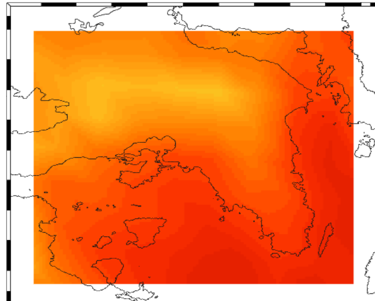
WRF 1x1km
